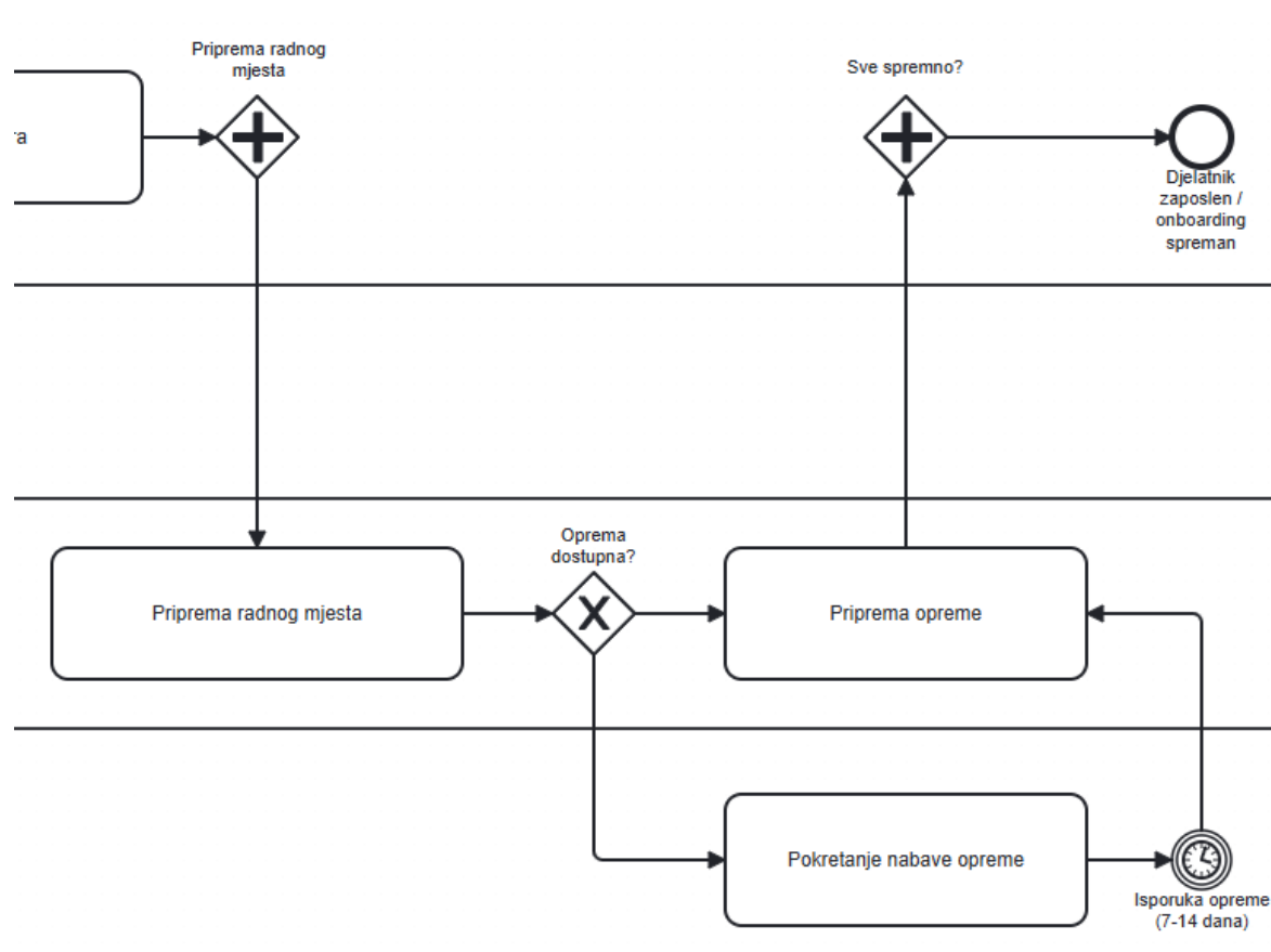
Slika 3: Paralelno izvođenje IT pripreme i nabave
